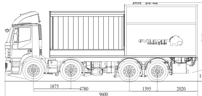
MSA 15.8 ALS PTO / MSA 15.5.3 ALS PTO
