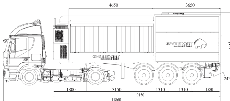
MSA 18.9 ALS / MSA 12.7.5 ALS / MSA 18.5.3 ALS
